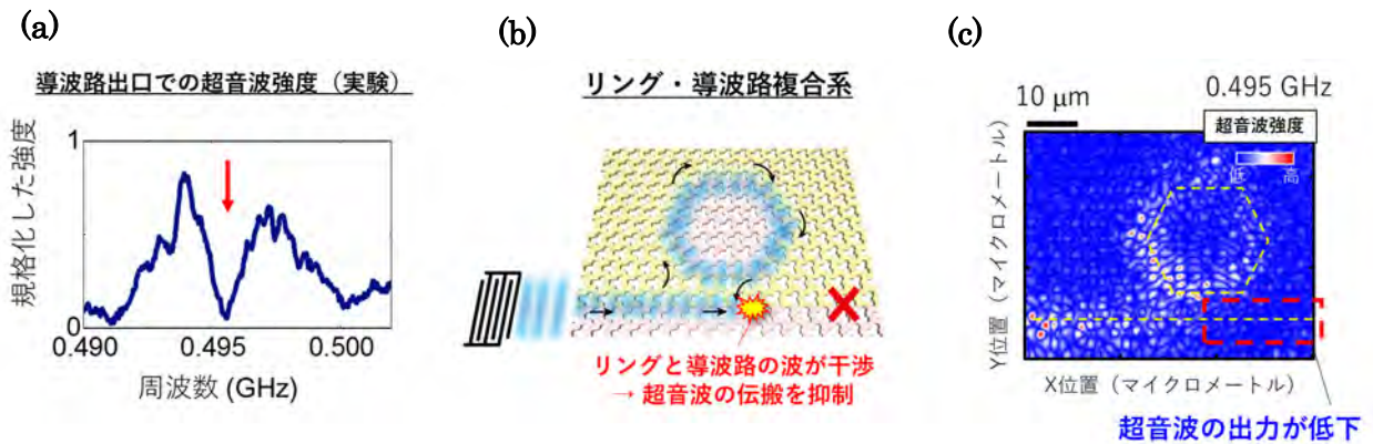
図4 : (a) トポロジカルリング・導波路複合系における導波路出力部での周波数応答。0.495 GHz 付近で出力が大きく低下するフィルタリング効果起きています (赤矢印)。(b) 超音波フィルタの原理を示した模式図。反射なく超音波がリング内を周回することで、リングと導波路の波が干渉し、導波路を進む超音波が抑制されます。(c) 周波数 0.495 GHz での超音波の空間伝搬の計測結果。超音波のフィルタリングにより、導波路における超音波の出力が大きく低下します。
