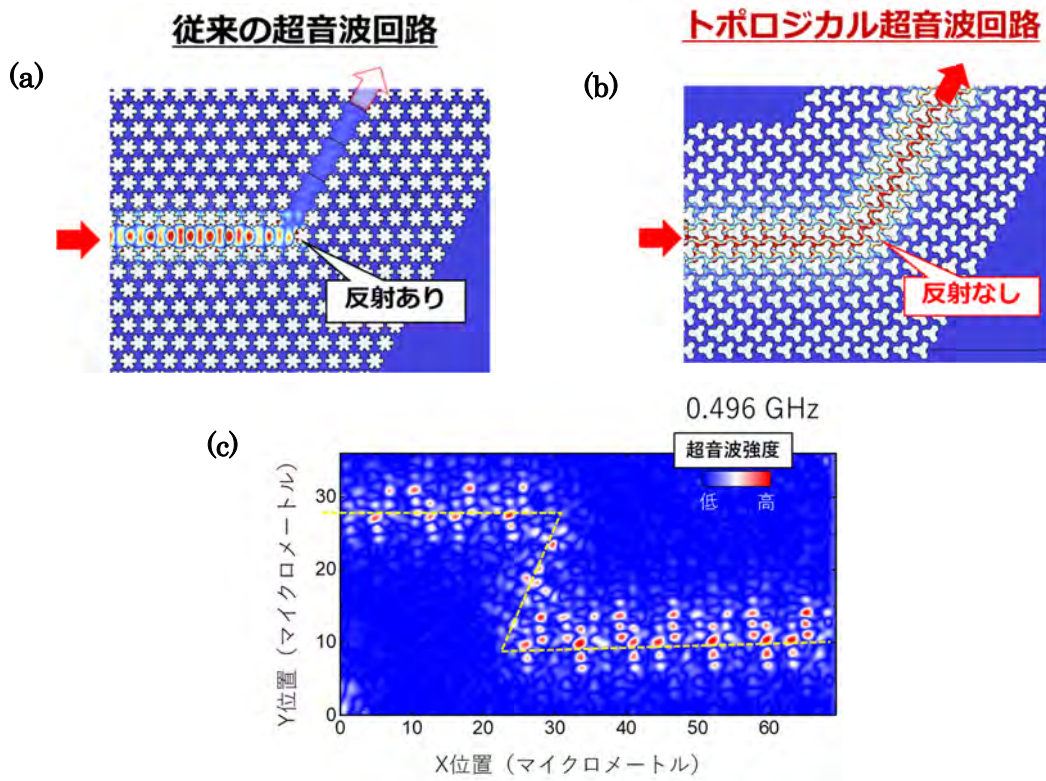
図3：従来の超音波回路 (a) とトポロジカル超音波回路 (b) をギガヘルツ超音波が伝搬する様子 (計算)。従来の回路は、周期孔の無い部分が導波路になっており、途中の120°折れ曲がった角で超音波は強い反射を受けます。一方で、トポロジカル回路では、反射を受けることなく滑らかに出口まで伝わります。両回路の周期穴間隔と入力した超音波の周波数は同程度であり、それぞれ4マイクロメートルと0.5GHzです。(c) アルファベットの”Z”のような形状をしたトポロジカル回路を伝わる超音波伝搬の測定結果。黄色の破線はエッジ部を示しています。
