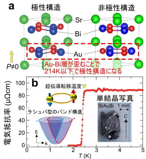
図1 SrAuBi の(a)結晶構造と(b)電気抵抗率での超伝導転移。極性構造ではBiの強いスピン軌道相互作用に由来したラッシュバ型のスピンスplitしたバンド構造が実現する。
