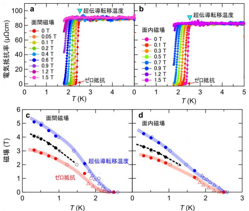
図2 SrAuBi の面間磁場(a)と面内磁場(b)での電気抵抗率での超伝導転移と面間磁場(c)と面内磁場(d)での超伝導臨界磁場
